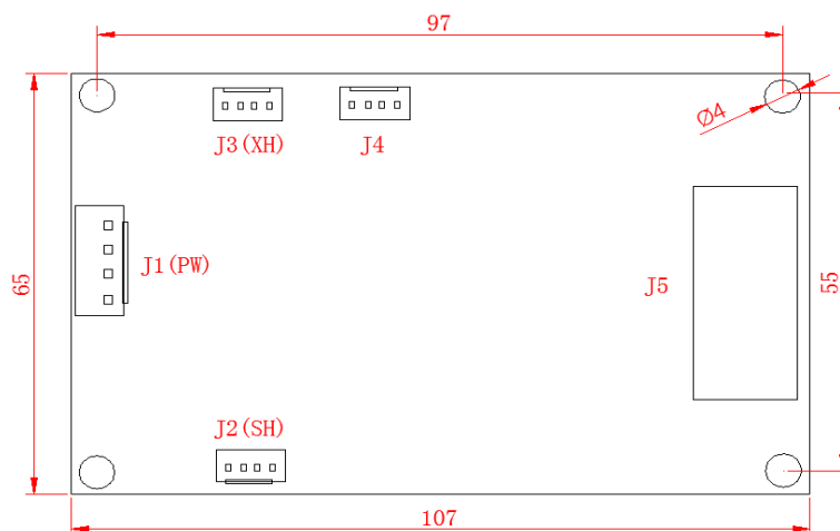
图 2.2 BL2000-HXJ-V9 尺寸图 (单位 mm)
